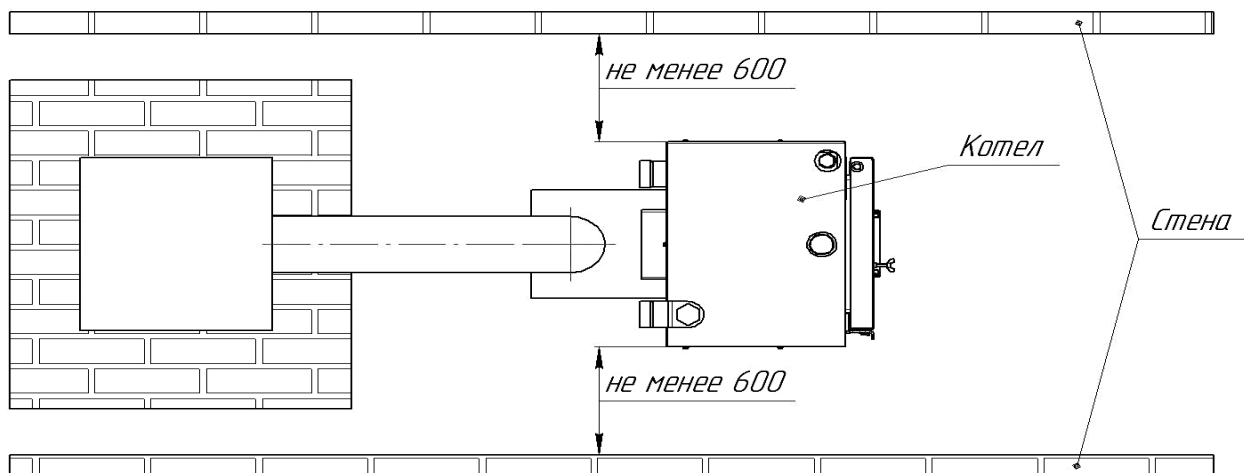
Рисунок 1 Схема размещения котлов КСТ-12,5; КСТ-16; КСТ-20
