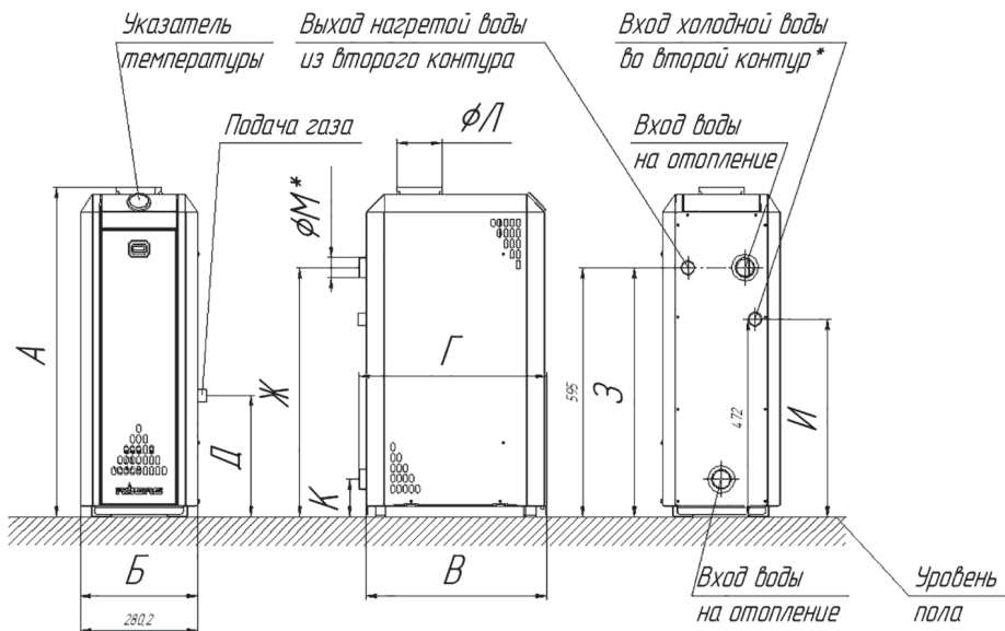
Рисунок 3. Общий вид котла
